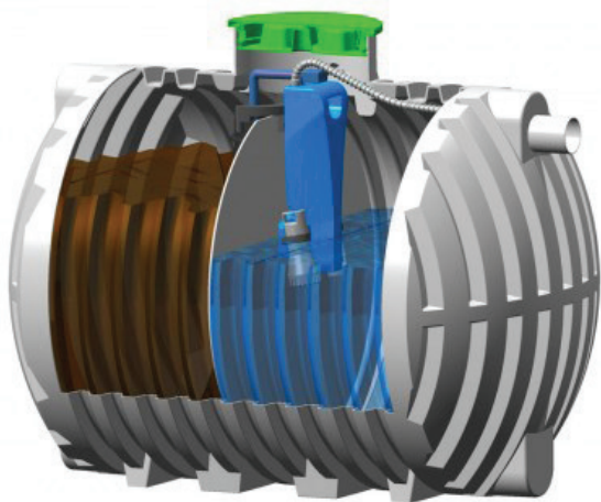
Komunalna čistilna naprava
